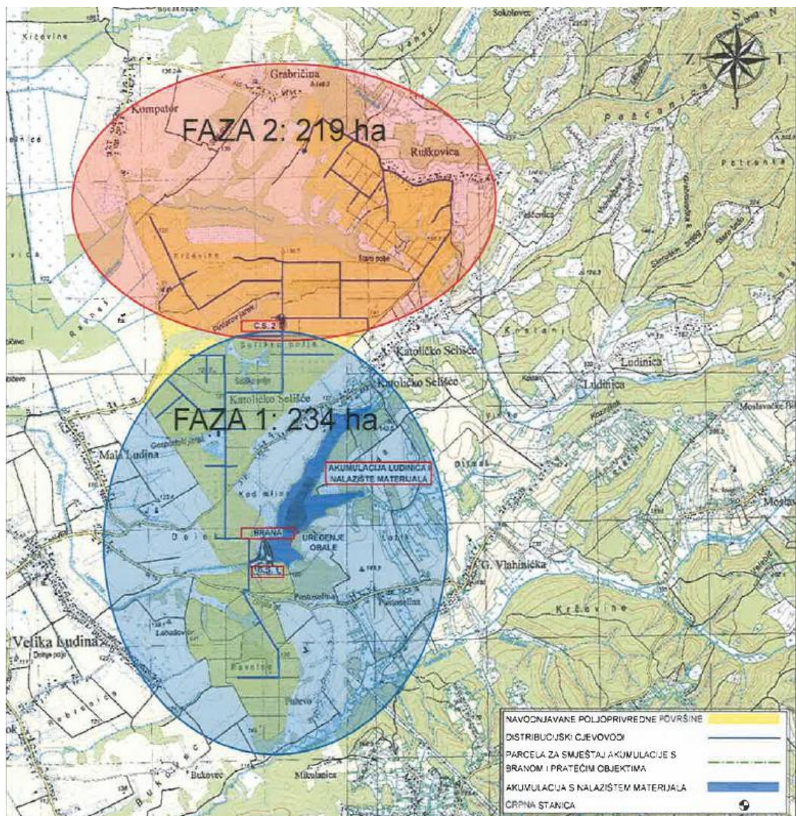
Slika 3. Tehničko rješenje faze gradnje SJN Velika Ludina predloženo od strane projektanata
